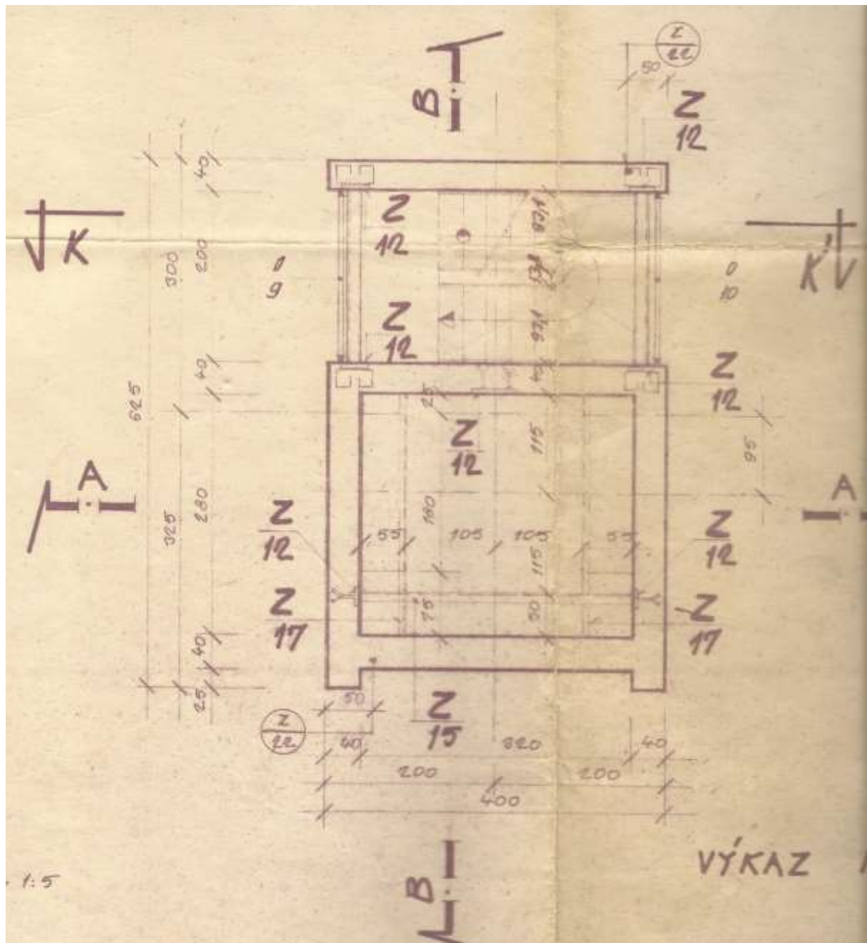
Obr.. Výťahová šachta VVnD typická v „drieku“ VVnD.
