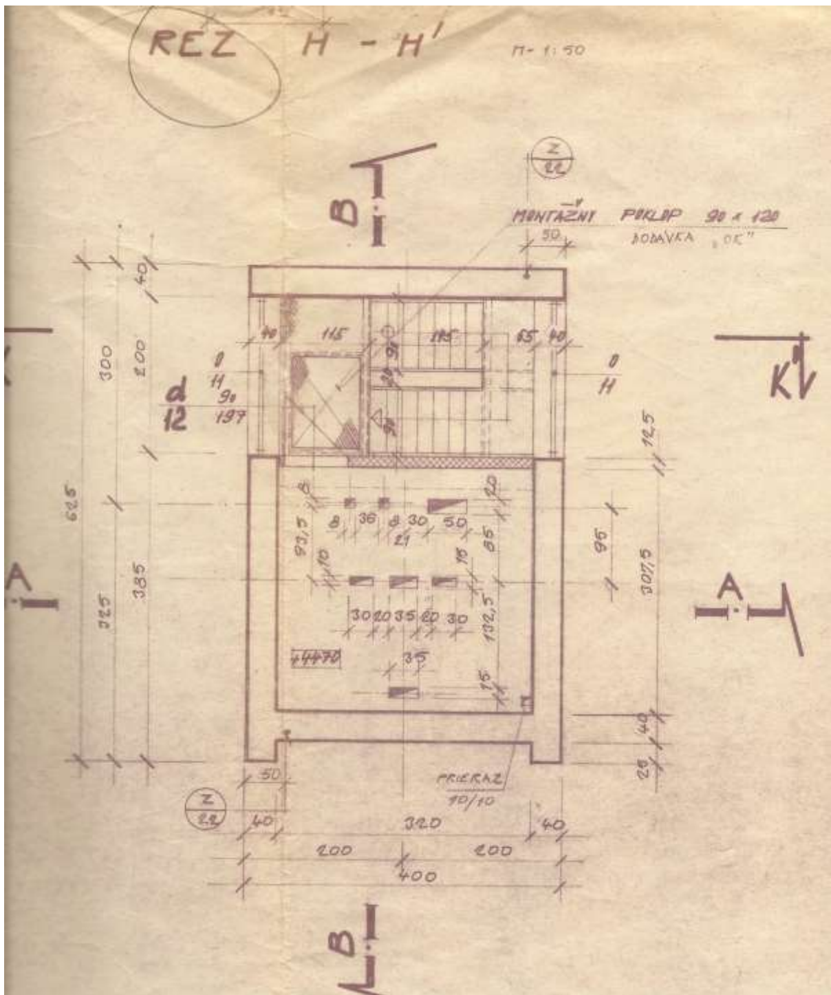
Obr.: Výtahová šachta na kóte +4470.
