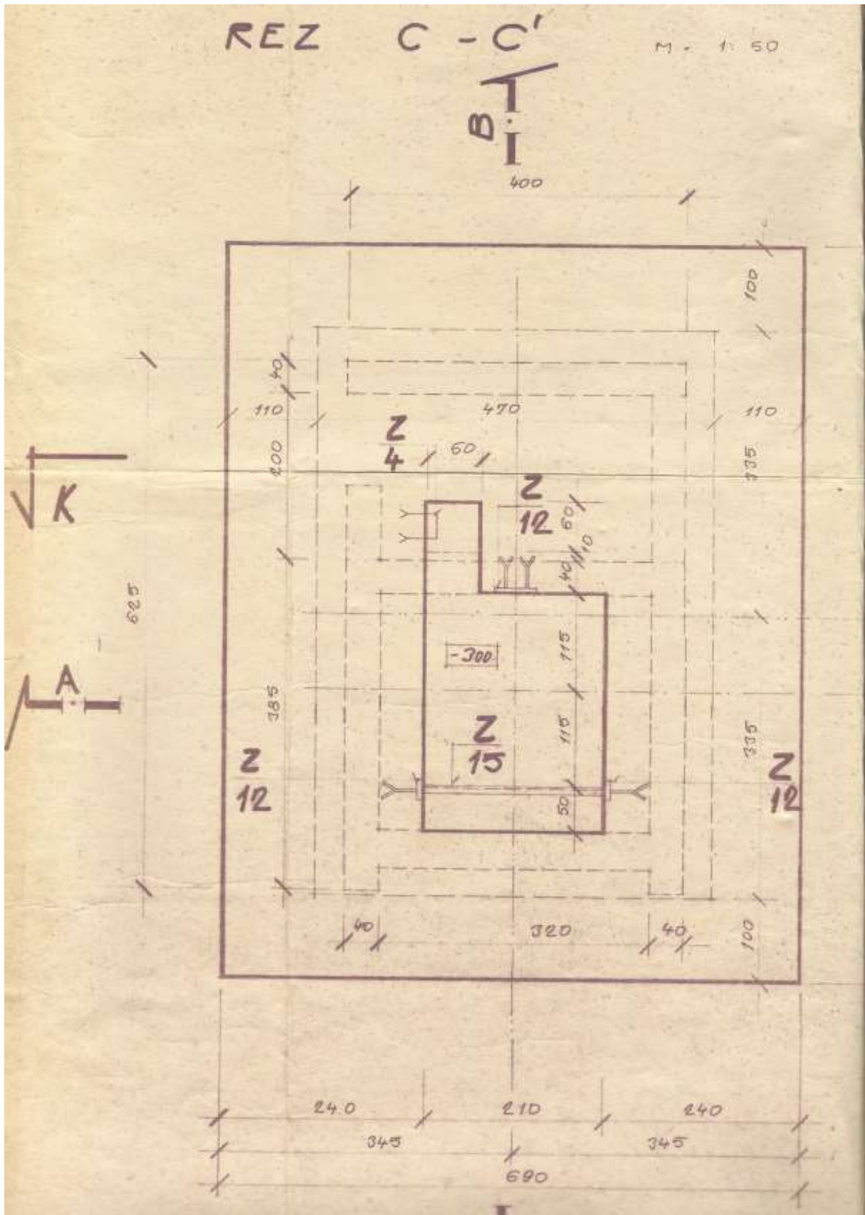
Obr.: Pôdorys na kóte -300.
