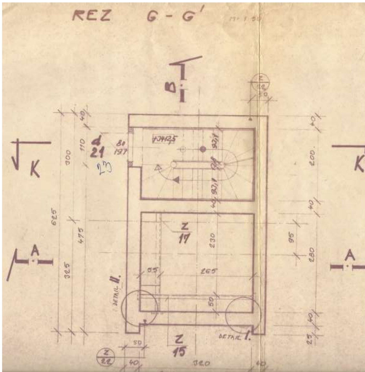
Obr.: Výtahová šachta na kóte +3425,5.
