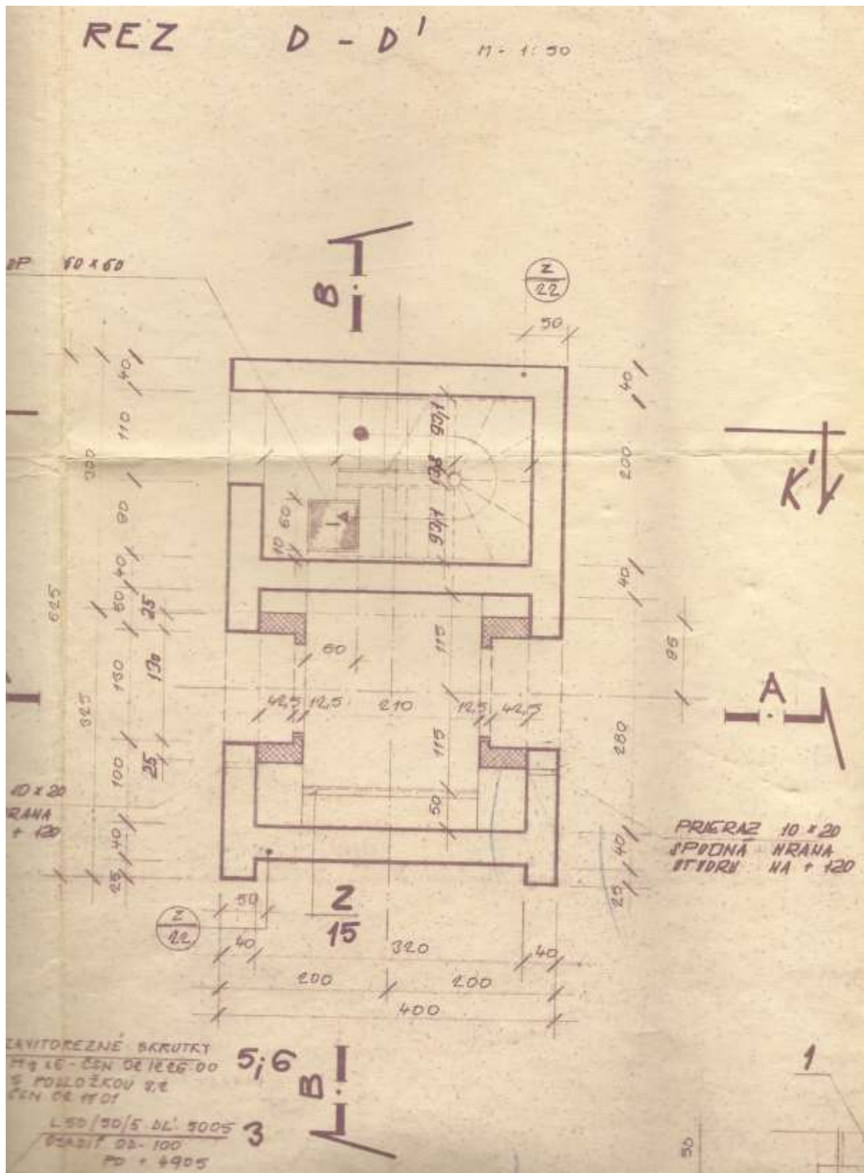
Obr.: Výřahová šachta VVnD na 1.N.P- obojstranný výstup a nástup
