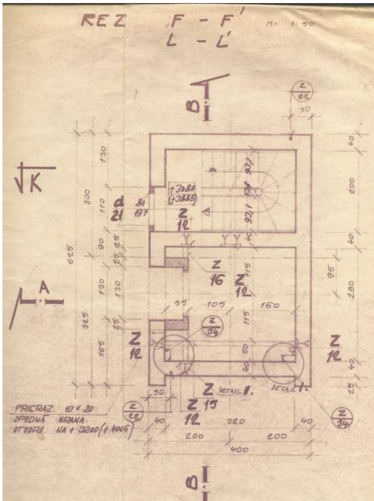
Obr.: Výťahová šachta na kupole VVnD – jednostranný výstup (kóta +2080 a +3885).
